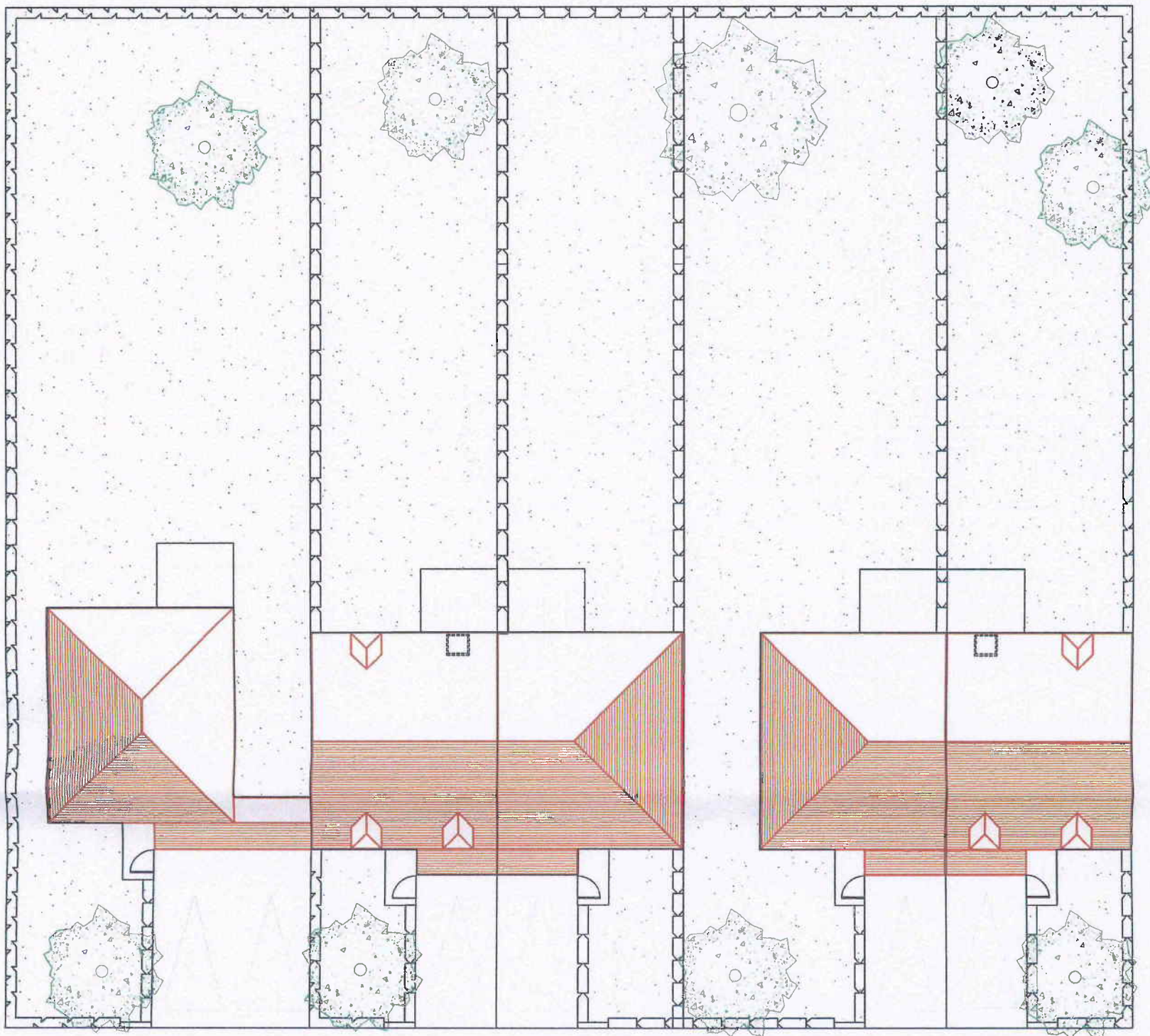
PLAN DE MASSE 1/200
